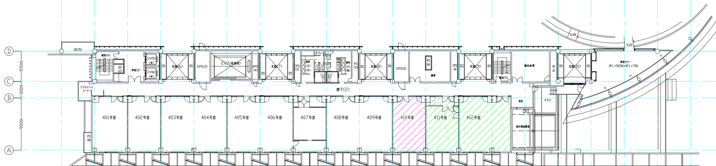
研究棟4階平面配置
